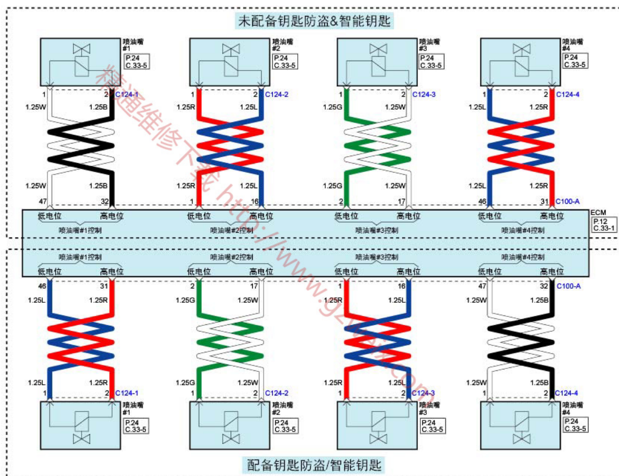
发动机控制系统(D4HB : R 2.2L VGT常规发动机)(6)
